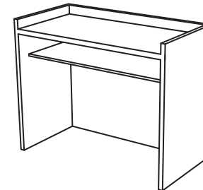
講演台 (800mm×1,600mm×H=1,000mm)
